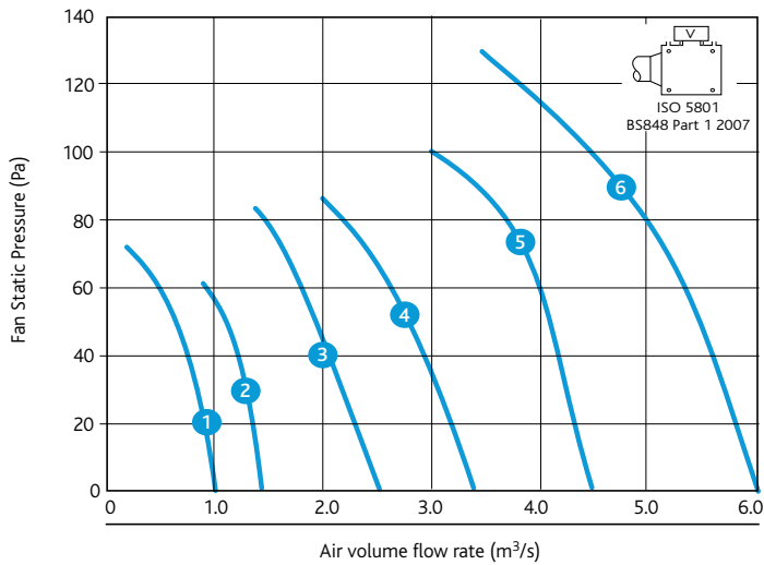
EZplate Axial Fan 8 Pole
